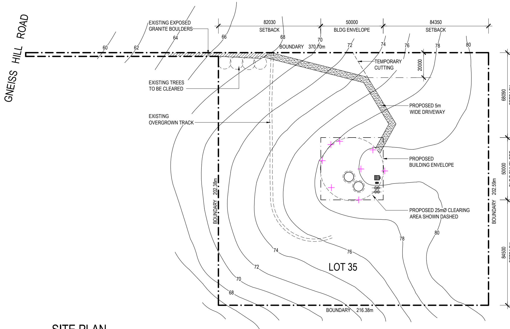
SITE PLAN SCALE 1:1500
